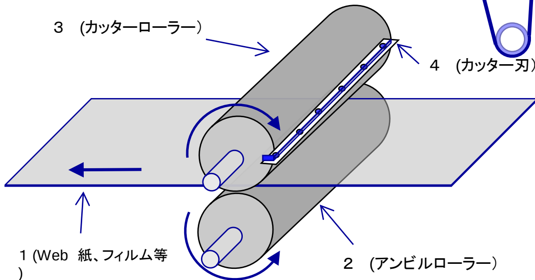
図1 従来のカッターローラーユニット
